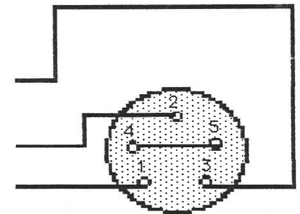
PRISE DIN MALE (agrandissement)
